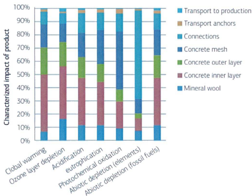
8. ábra: ECOSANDWICH környezeti hatásának értékelése
