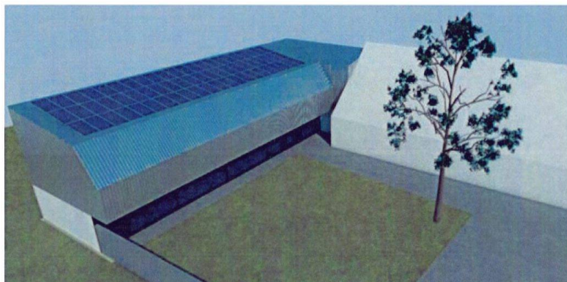
22. ábra: Napelemtelepítés a Deák Ház tetőszerkezetére - látványterv
