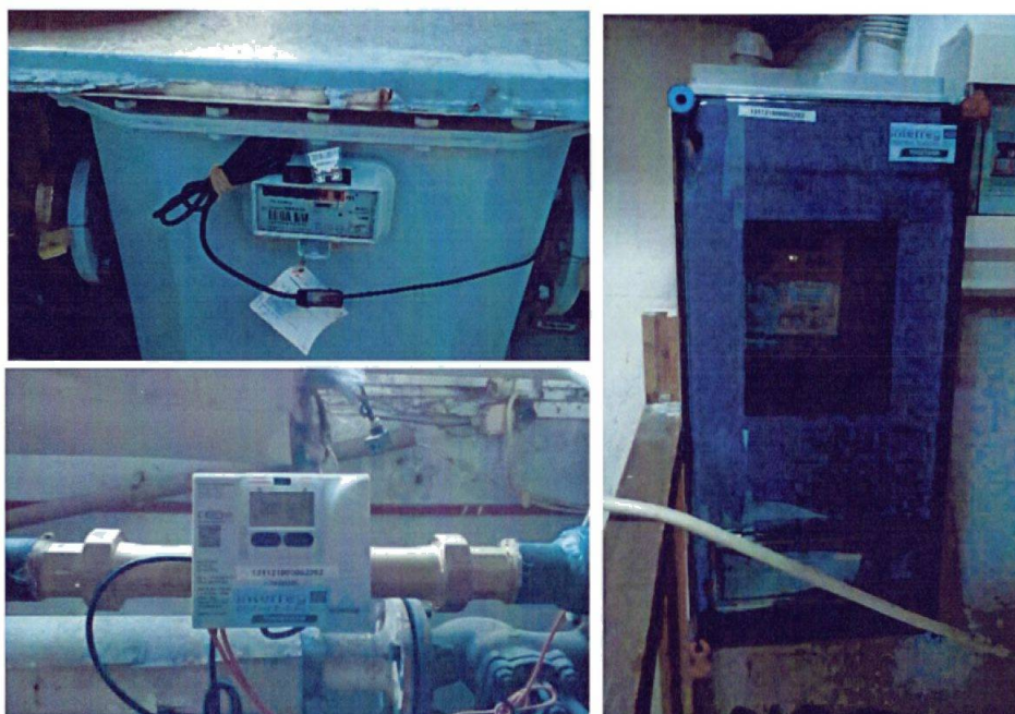
18. ábra: Gázóra kommunikációs jeladóval, hőmennyiség mérő, villamos okos mérő
