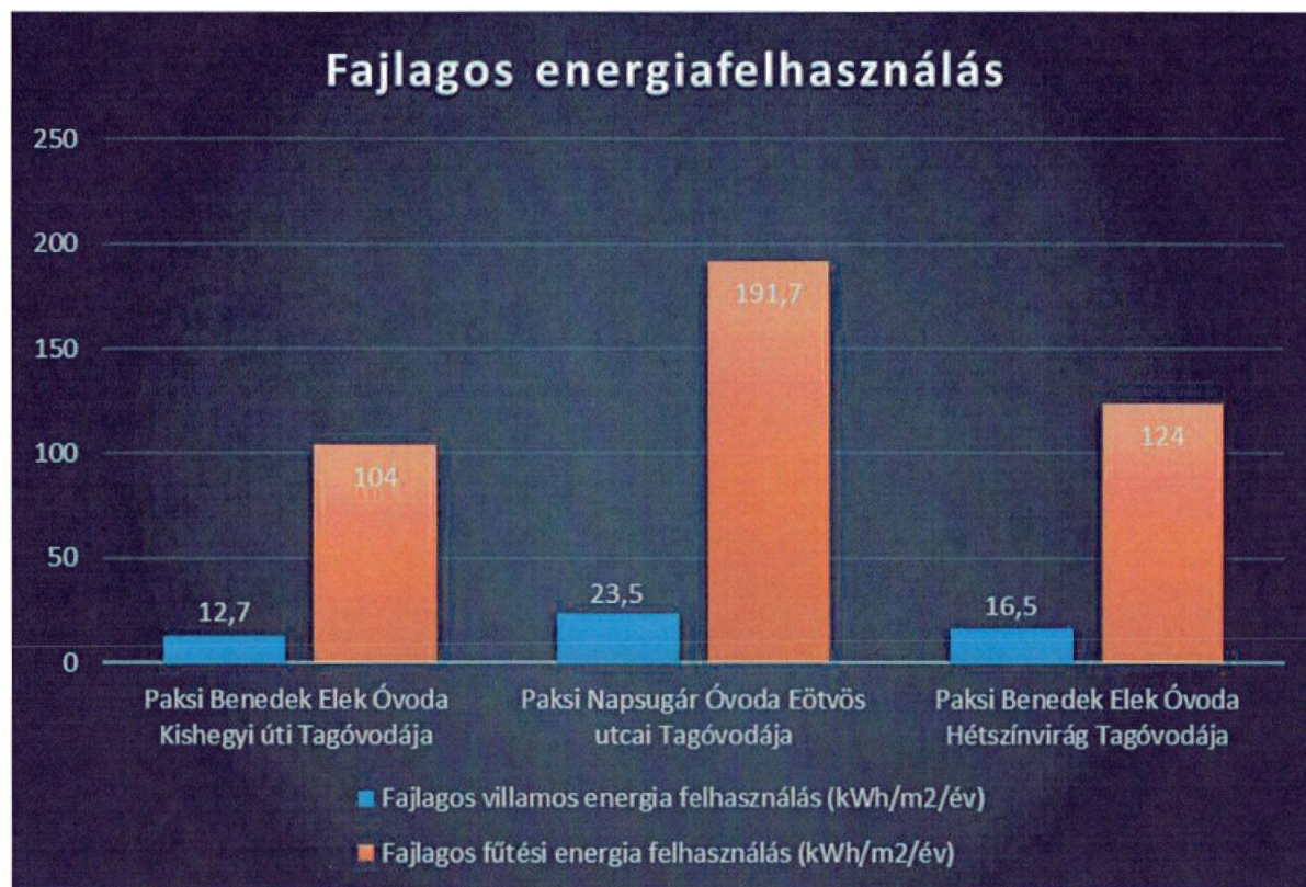
5. ábra: Az óvodaépületek fajlagos energiafogyasztásának összevetése
