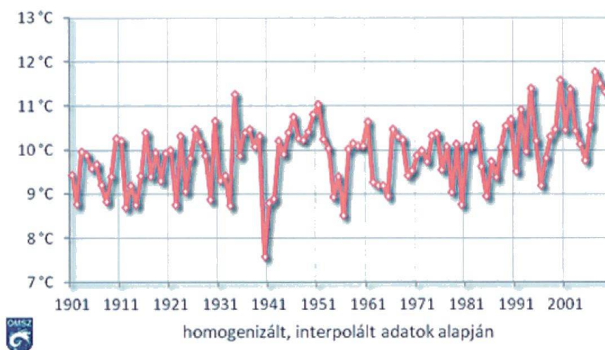
6. ábra: Országos évi középhőmérsékletek (1901-2009) [Forrás: MET]
